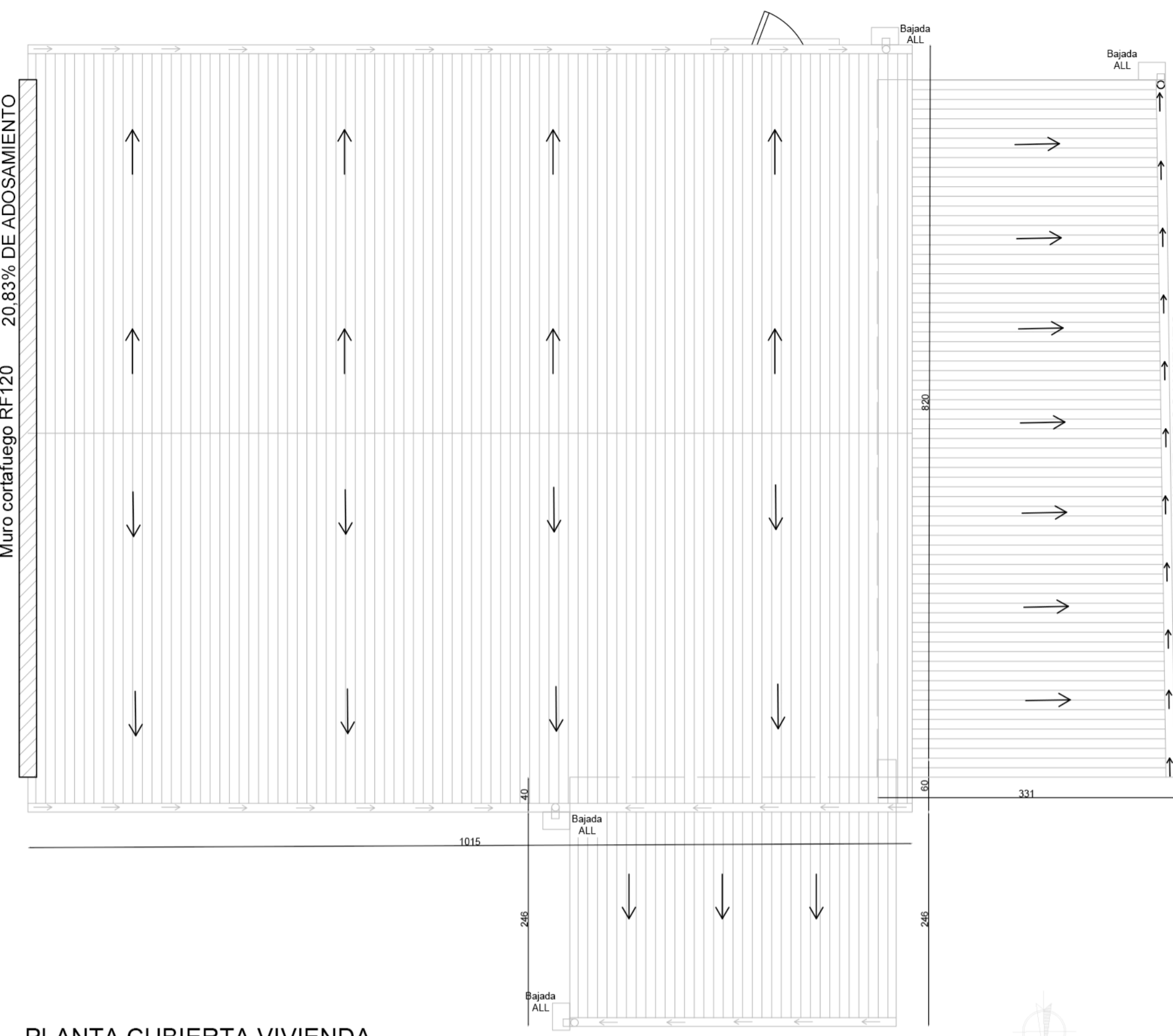
PLANTA CUBIERTA VIVIENDA ESC. 1/50
